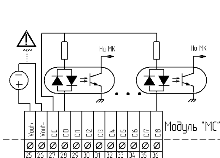
Рисунок 12. Упрощенная электрическая принципиальная схема цифровых входов МС. DIC – общая клемма, D i – вход двунаправленного оптрона, Vout+ Vout- - выходы внутреннего источника напряжения цифровых входов.
