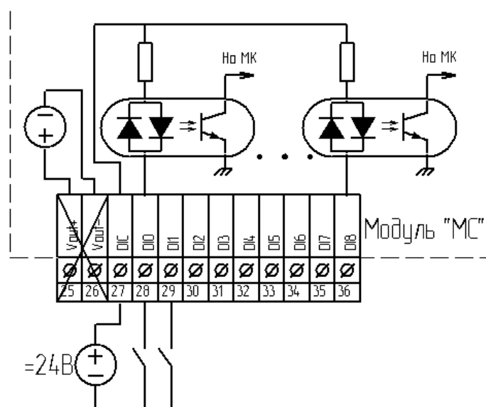
Рисунок 14. Пример подключения датчиков типа «сухой контакт» с питанием от внешнего источника напряжения
