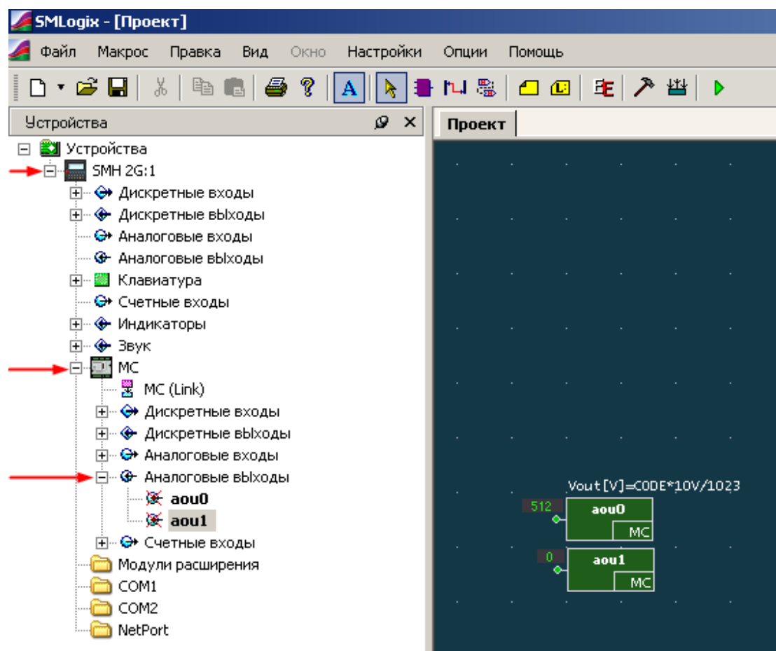
Рисунок 29. Использование аналоговых выходов MC.
