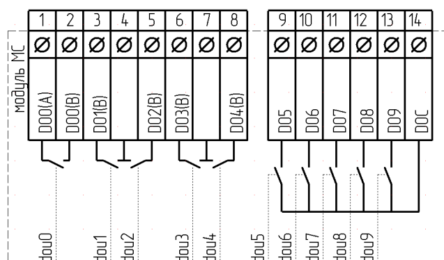
Рисунок 191. Использование цифровых выходов.
