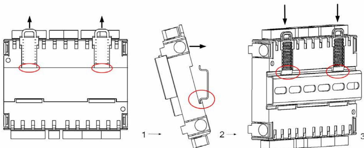
Рисунок 4. Установка МС на DIN-рейку
