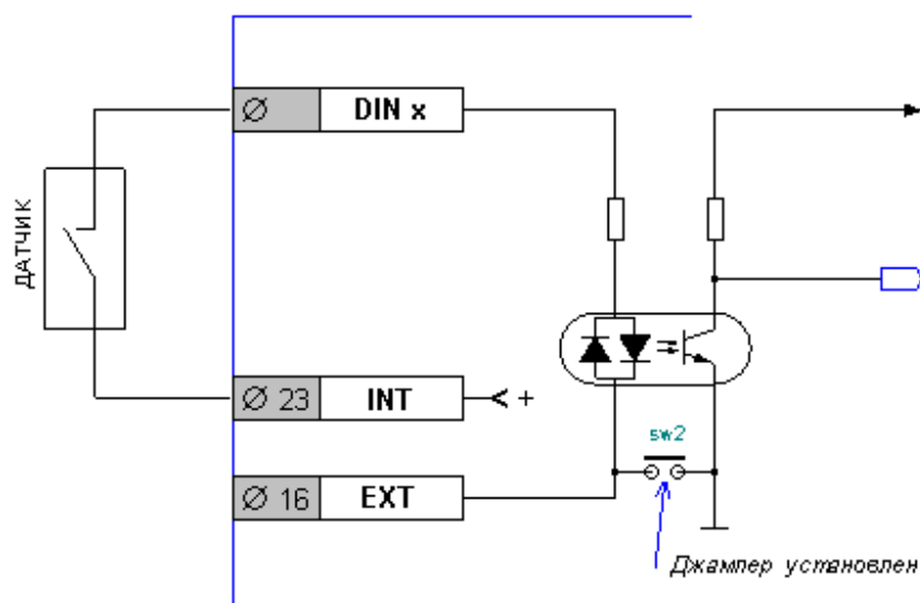
Рисунок 32. Схема (условная) дискретного входа
