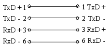
Прямое соединение “Straight-through”
