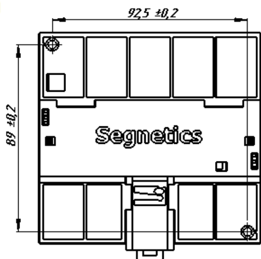
Рисунок 15. Монтажные размеры отверстий
