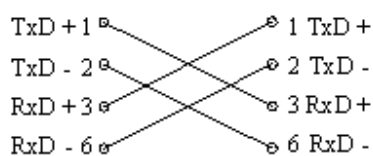
Перекрестное соединение “Crossover”
