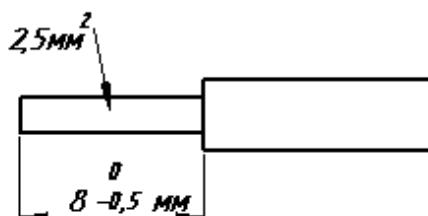
Рисунок 27. Заделка провода
