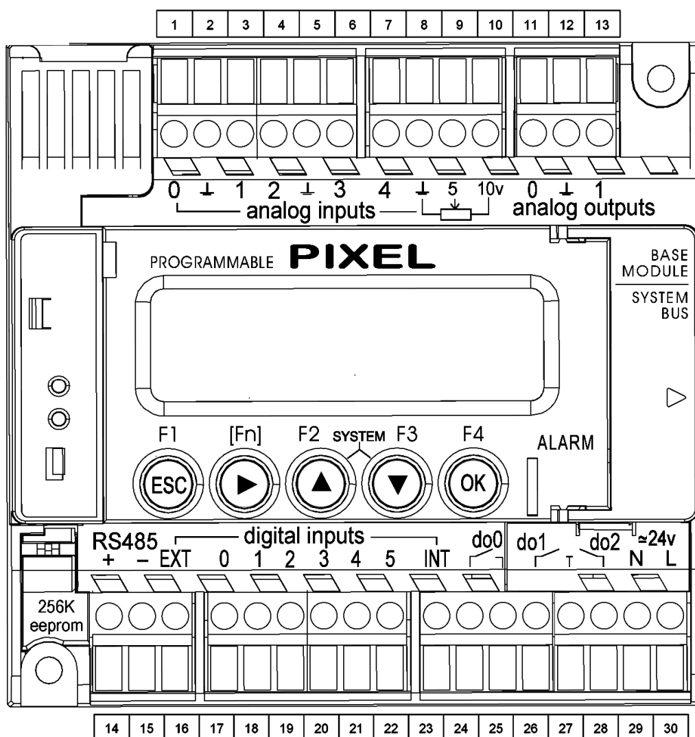
Рисунок 17. Маркировка клемм контроллеров Pixel – xxx1-xx-x и Pixel – xxx2-xx-x
