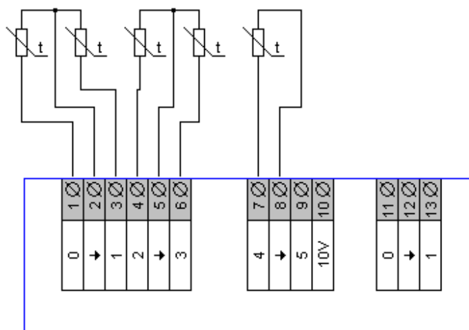
Рисунок 50. Подключение термосопротивлений
