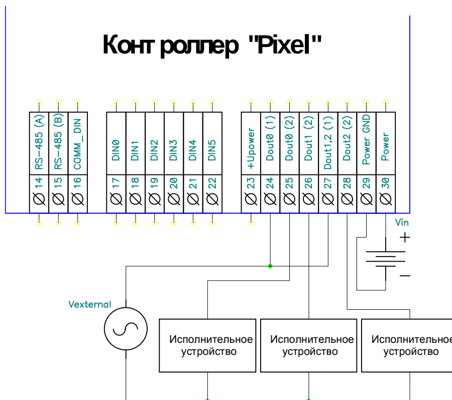
Схема подключения исполнительных устройств к выходам
