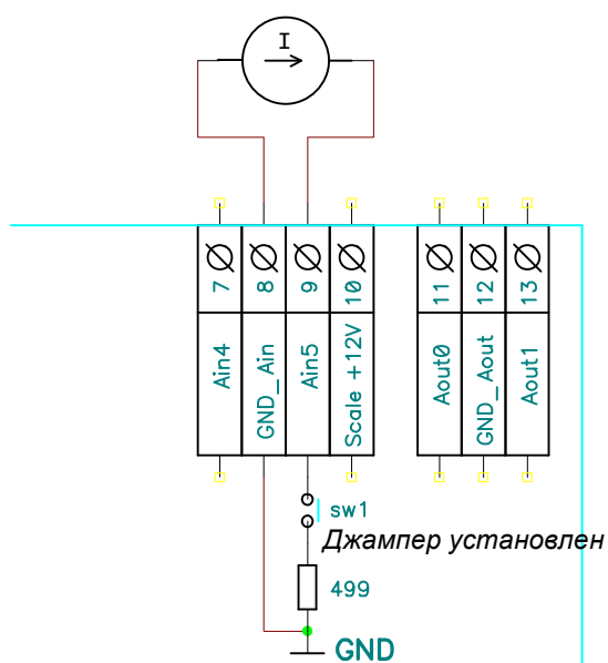
Контроллер "Pixel"
