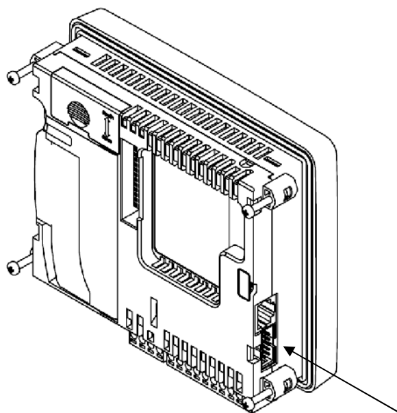
Разъем для подключения модулей расширения
